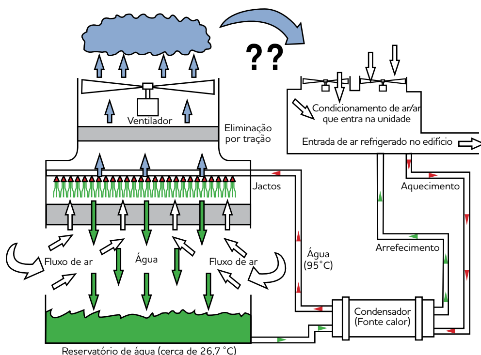
Figura 5: Perigo associado à proximidade de torre de arrefecimento e de tomadas de ar no edifício
