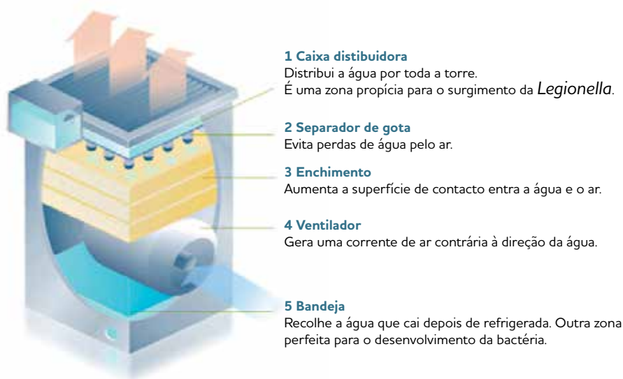
Figura 6: Descrição das partes de uma instalação
