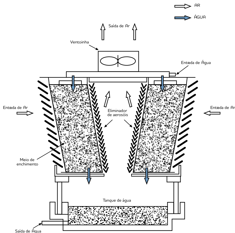
Figura 7: Torre de arrefecimento ou refrigeração para edifícios de grande dimensão (Department of Human Services, Guidelines for the control of Legionnaires' Disease, Victoria Melbourne Australia)
