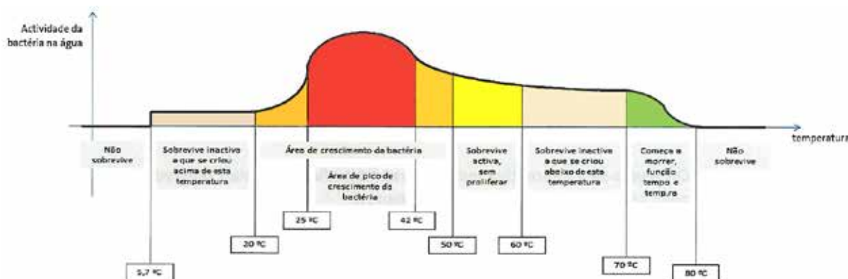
Figura 13: Atividade da Legionella na água a diferentes temperaturas (Fonte: Grundfos Alldos Dosing & Disinfection. "Guidelines for combating Legionella with Oxiperm Pro chlorine dioxide systems" www.grundfosalldos.com )
